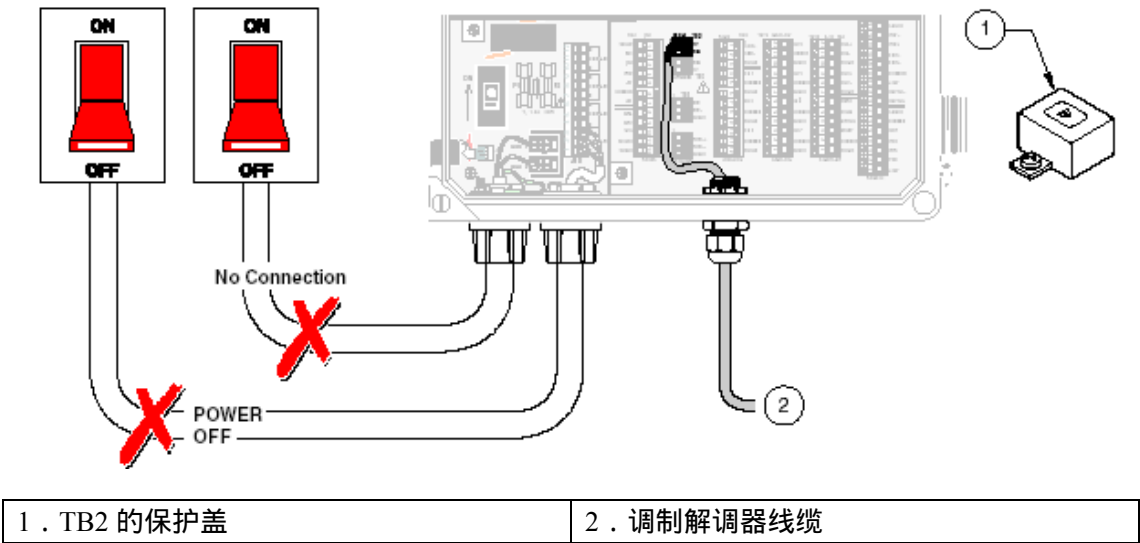
图 20 调制解调器接线连接
